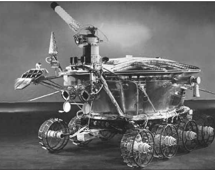
Луноход-1 — первый лунный самоходный аппарат. Он был доставлен на поверхность Луны 17 ноября 1970 г. советской межпланетной станцией Луна-17.
