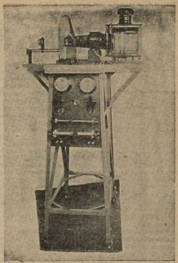
Телевизионная установка
