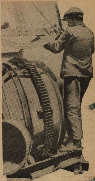
Установка бетономешалки
