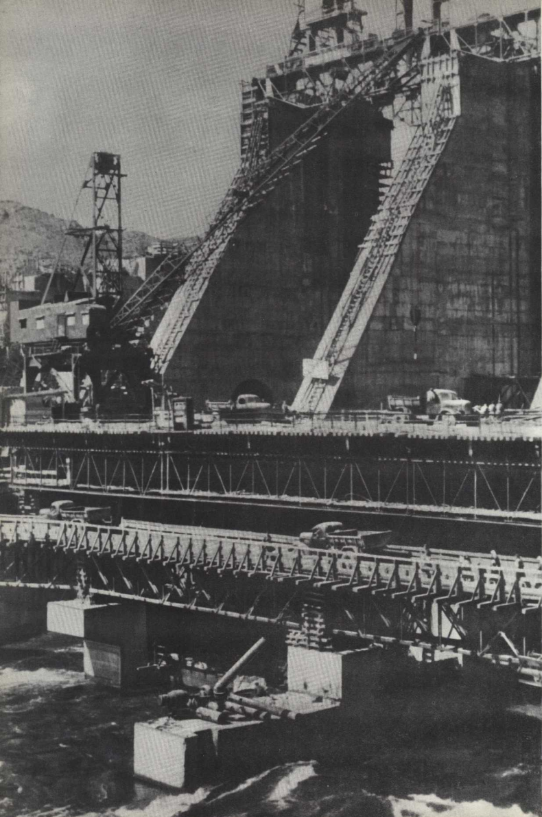
Усть-Наменгорская ГЭС на реке Иртыше; водосливная часть плотины.
