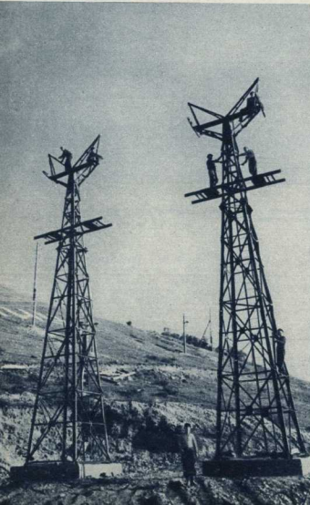
Установка металлических мачт-опор на горе Могутовой для подвесной канатной дороги.
