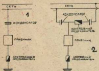
1. Прием на осветительную сеть при включении на один провод. 2. Схема приема на осветительную сеть с клеммой оба провода.
