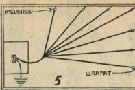
Верхообразная комнатная антенна.
