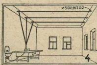
Треугольная комнатная антенна.
