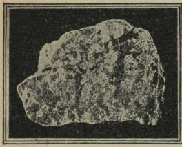
Фотография снятого при дневном свете кусочка урановой смолки, из которой добывается радий.
