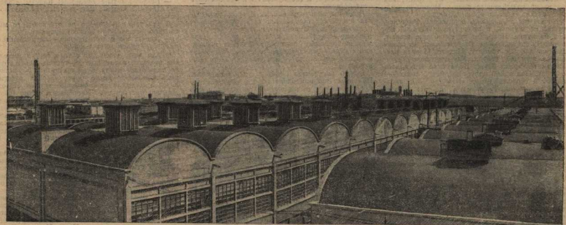
К XV Октябрю построен электролитный цех — гигант алюминиевого завода Днепрокомбината
