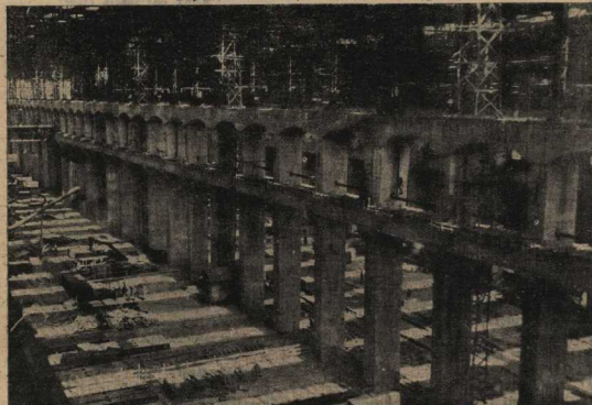
Строящиеся цехи огромного завода турбостроения по своей величине превосходят самые большие цехи крупнейших заводов. Завод строит в Харькове — столице советской Украины
