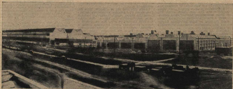
Вслед за Сталинградским и Харьковским в этом году вступает в строй Челябинский тракторный завод. Ты видишь на снимке механосборочный и инструментальный цехи, которые начали работать еще в феврале.
