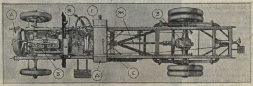
ОБЩИЙ ВИД АВТОМОБИЛЬНОЙ РАМЫ С МОТОРОМ: а) радиатор; б) мотор; в) конус; г) коробка скоростей; д) бензиновый бак; е) глушитель; ж) вал мотора, идущий к шестерням; з) концы передаточного вращающего вала на ось колес.
