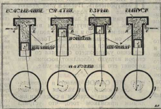
ВВЕРХУ — общий вид автомобильного двигателя внутреннего сгорания. В СЕРЕДИНЕ — СХЕМА РАБОТЫ ЧЕТЫРЕХТАКТНОГО ДВИГАТЕЛЯ ВНУТРЕННЕГО СГОРАНИЯ: (рис. 1): а) всасывание горючей смеси из карбюратора; б) сжатие ее поршнем, идущим вверх; в) взрыв смеси от закрывающегося клапана и от быстрого движения и падения поршня вниз; ВНИЗУ СЛЕВА — УСТРОЙСТВО КЛУСА, который позволяет развить, работающий мотор с переднего на колеса. (рис. 2); Нижняя часть — маховик колеса, сидящий на полу двигателя или движущийся по нему; Т — сцепление безобитающего с осью, отбрасывающего вперед барабанчик и, насаженный на ось, переключает передачи к колесам. ВНИЗУ СПРАВА — Тип легкой и дешевой амортизации, к которой совершенно не применима у американских фермеров желтую сталь.
