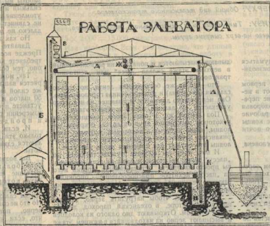
СХЕМА РАБОТЫ ЭЛЕВАТОРА: а) приемный коловдез в который спускается зерно из вагона; б) норья, поднимающая зерно в верхний этаж, откуда оно попадает на транспортер II, загружающий его в место хранения. Для выгрузки открывается дно нужного отделения и зерно из него попадает на транспортер 3, доставляющий в коловдез II, и норья II поднимается к трубе II, опущенной в трюм парохода.
