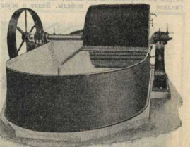
ОБЩИЙ ВИД ГОЛЛАНДЕРА: Он превращает грязное тряпье в бумажную полумассу, состоящую из отдельных головок с распущенными концами.
