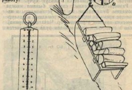
Пружинные весы А, прикрепленные к веревке, покажут силу пружины, которая тянет санки вперед, когда человек тянет их.
