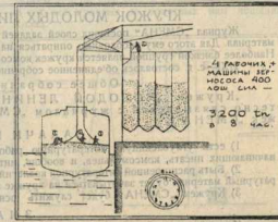
СХЕМА ПНЕВМАТИЧЕСКОЙ ВЫГРУЗКИ: 30.000 пудов на человека в 8-час. раб. день.
