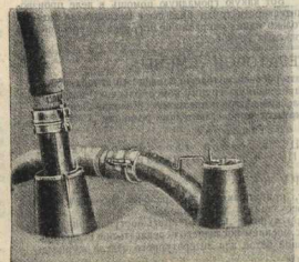
Концы всасывающей трубы, опущенной в трюм.
