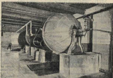
ШАРОВЫЕ КОТЛЫ ДЛЯ ВАРКИ ТРЯПЬЯ: после режки из тряпья надо убавить всю грязь и краску. Для этого его вымачивают в растворе едкого натра или извести.
