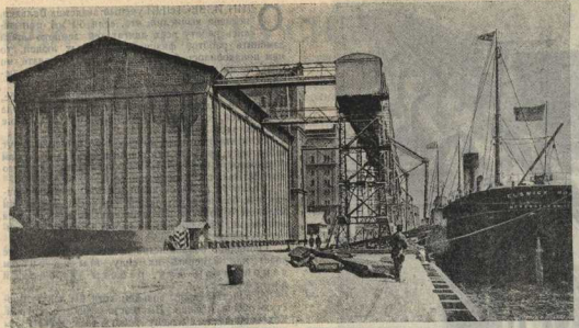
ОБЩИЙ ВИД ЭЛЕВАТОРА во время на.руки парохода зерном. На снимке видна труба, по которой зерно спускается в трюм.
