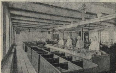
СОРТИРОВКА ТРЯПЬЯ: прежде, чем пустить тряпье в обработку его раскортнривают по ряду «келлан»: льняную тряпку к льняной, хлопковую к хлопковой.
