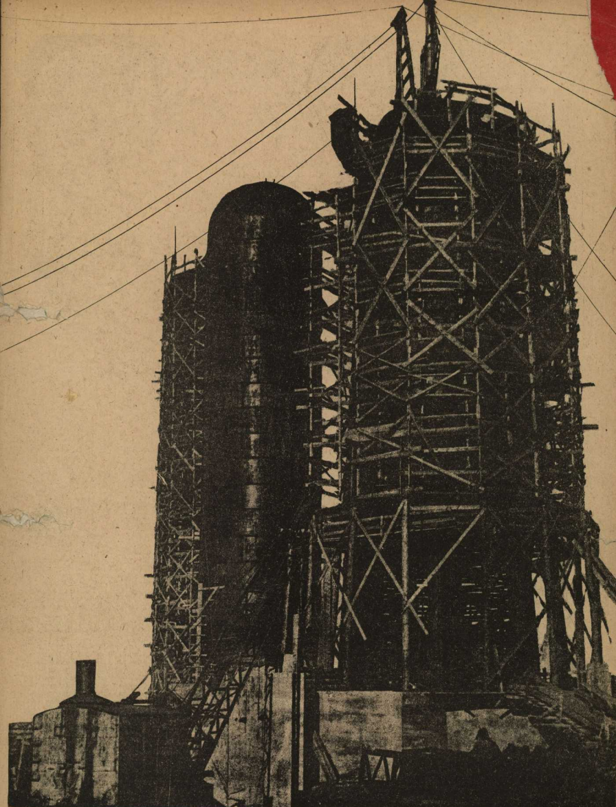
на снимке — знакомые очертания домы, это домна № 2 кузнецкого металлургического завода, сейчас на ней заканчивается установка газопровода.
