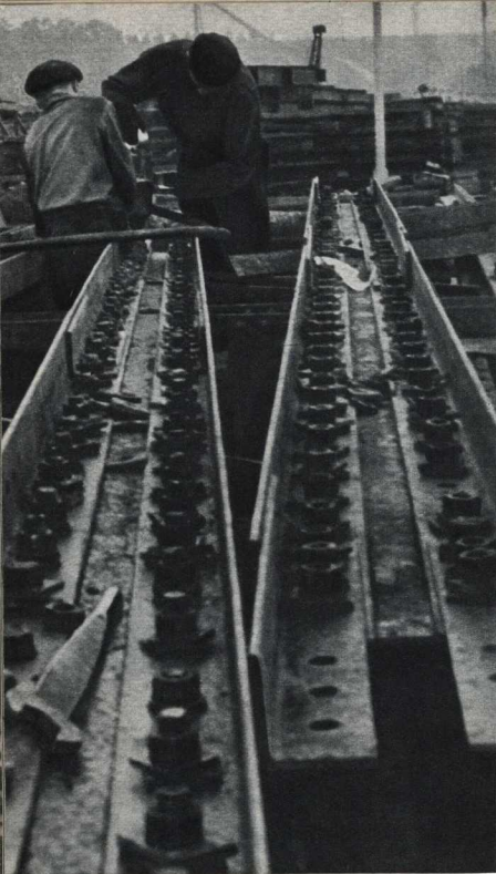
Здесь собирают специальные металлические опоры, которые будут под- держивать арку моста при транспортировке его на понтонах.
