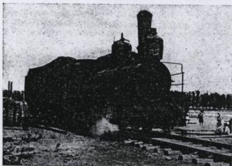
Недавно закончен северный участок ж.-д. магистрали между Сибирью и Туркестаном. На фото — первые паровозы на левобережье Иртыша.
