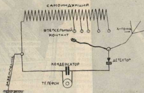
Рис. 2. Схема соединения приемника.
