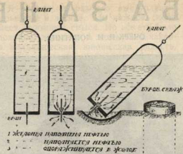
Добытие нефти из буровой скважины с помощью желонки.
