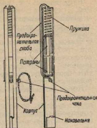
Металлический воспламенитель
