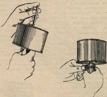
Ручная противотанковая граната ударного действия
