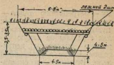
Ловушка для танков
