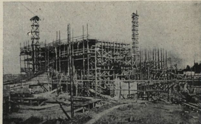
В Белоруссии (среди торфяных болот строится Осиновская электростанция (Осинстрой) мощностью в 20000 киловатт. На фото—сооружение главного корпуса.
