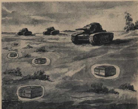
Противотанковые мины расставлял на дорогах, по которым скорее пройдут вражеские машины. Расставлять их надо в шахматном порядке, чтобы фашистский танк никак не сумел их избежать. Мины не засыпаны сверху. Верхняя крышка корпуса мины должна на 1–1,5 сантиметра возвышаться над уровнем земли.
