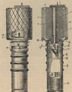
Граната образца 1933 года
