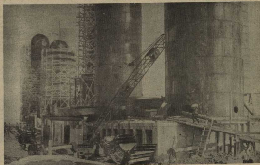
Заканчивается монтаж на кулерах доменного цеха
