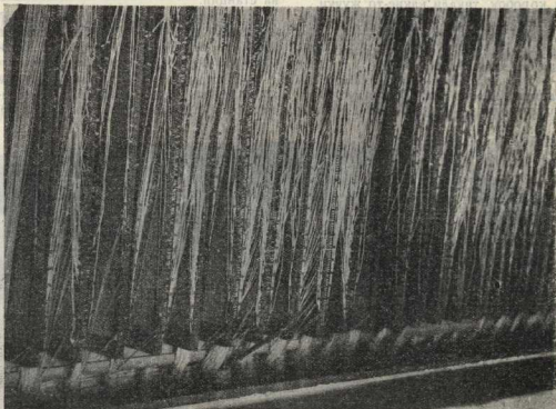
«КРОСС» — сердце телефонной станции, — зал, в который сходятся все провода телефонной сети. Каждый абонент имеет здесь свой отдельный провод.
