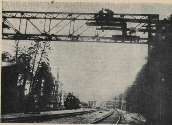
Установка контрольных счетчиков на электрифицируемом участке Северных железных дорог.
