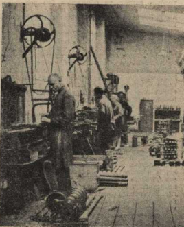
Новый токарный цех завода «Буровая техника» (б. Виноградова) встречает простором и светом
