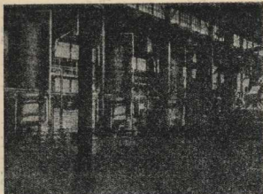
ЭДЖЕВУДСКИЙ АРСЕНАЛ: внутренний вид завода хлор-никринов, применяемого для изготовления артиллерийских снарядов. За несколько лет этот завод успел выработать около 140.000 пудов хлор-никрина, при чем эта цифра, как говорит официальный отчет, — не показывает максимальной производительности завода.
