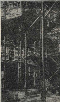
РЕАКТОР ЛЕВИНШТЕЙНА, установленный в Эджевудском Арсенале для приготовления горючего газа. С помощью этой установки Эджевуд способен выпускать до 2400 пудов газа в сутки.
