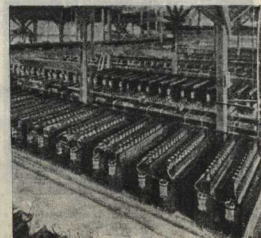
ВНИЗУ: ЭДЖЕВУДСКИЙ АРСЕНАЛ: внутренний вид одного из двух зданий с батареями Нельсона для выработки хлора в лабораторическом туман. Каждое здание имеет 541 фут длины и разделено на четыре вполне самостоятельных по оборудованию отделения; вертикальность всех искривлений отделений увеличивает боевую производительность хлора в сутки.
