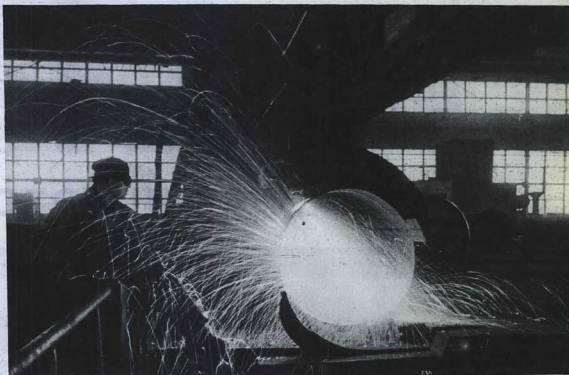
Огромный стан для сварки крупно-размерных труб кажется совсем небольшим в эскизном цехе Ново-Московского завода.
