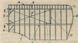
Крыло злера в собранном виде (рис. 15): А—ребро атаки, В—промежуточное ребро обшивки, С—задний ложкераон, D—руль злера, E—уловка распорки, F—коробчатая нервюра, G—место присоединения к фюзеляжу, H—нервюра, I—ребро шхона, L—внутренняя распорка из стальной проволоки, M—распорная труба.
