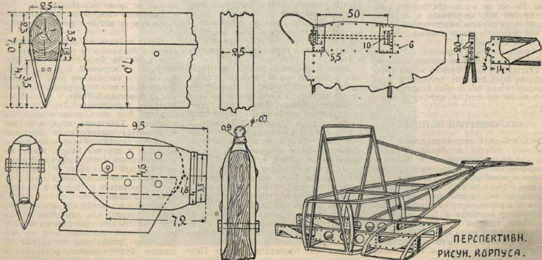
СПРАВА ВНИЗУ (рис. 16): перспективный вид фюзеляжа до обшивки его фанерой.
