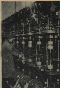
НОВЫЕ ПРОИЗВОДСТВА. Завод «Совнабель» приступил к изготовлению нового типа кордельного кабеля для одновременной передачи телефонного разговора, телеграфа и изображений на расстоянии. До последнего времени этот кабель ввозился из-за границы.
