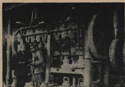
СТРОИТЕЛЬСТВО УРАЛА. Механизированный кирпичный завод, производительностью 50 млн. кирпича в год.
