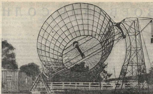
Солнечный двигатель Эриксона в Лос-Анжелесе (Калифорния С.-А. С. Ш.). Возвзает зеркало, диаметром 10 метров, вращается на оси вслед за солнцем. Оно состоит из 1788 маленьких плоских зеркал, отражающих солнечные лучи на асбестовый медный котел в виде трубы, укрепленный в конусе зеркала. Вся установка приводит в действие 9-ми силую паровую машину низкого давления.
