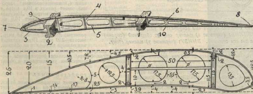
Нервура крыла (ПОПЕРЕЧН. РАЗР.) 1/5
