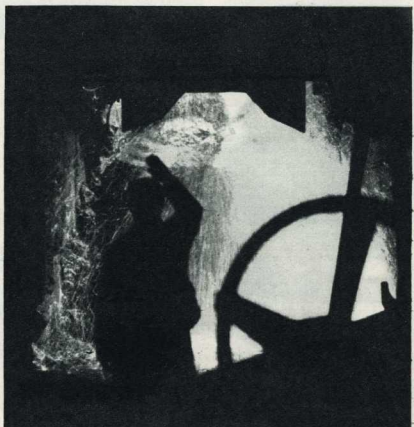
Бессемеровский чех. В конвертер подан кислород, продувана мугуна началась...
