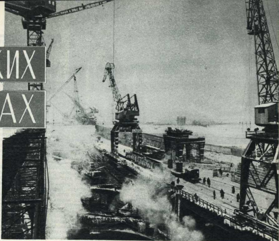
Монтажные работы на стройке Куйбышевской ГЭС.
