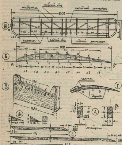
СЛЕВА — УСТРОЙСТВО КРЫЛА (черт. 3): а — скелет ось о крыла; б — детали нервура; в — устройство шаблона для изготовления нервура; г — внешний вид нервура; д — разрез переднего (слева) и заднего (справа) ложенерона; СПРАВО. ДЕТАЛИ УСТРОЙСТВА КРЫЛА (черт. 4): а — конюльда часть ложенерона; б — боковой ободок крыла; в — общий вид собранного крыла.
