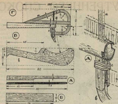
РУЛЬ НАПРАВЛЕНИЯ (черт. 6): а—вертикальная стойка служащая осью руля, б—скрепляющая пластинки, в—костыль, г—устройство ручки, д—деталь прикрепления к острию.
