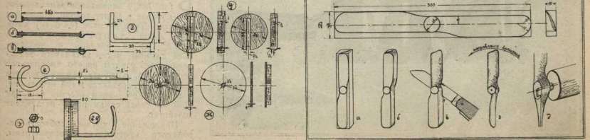
СПРАВА.—ПРОПЕЛЛЕР (черт. 8): последовательность его изготовления и деталь укрепления на оси. СПЛЕВА!—РЕЗИНОВЫЙ МОТОР (черт. 9): а, б и в—три способа укрепления резиновой нити, г—неподвижный крючок, д—деталь его устанювки, ед—ось пропеллера, ж и з—детали укрепления ее.
