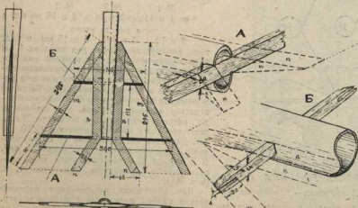
СЛЕВА — РУЛЬ ВЫСОТЫ (черт. 5): а и б — передняя и задняя боковые планки, составляющие остов руля высоты. СПРАВА — УСТРОЙСТВО КРЫЛА (черт. 7): а — от двух с лыж; б в — желуди насадки; г — распорка шасси; д — железная ось для колес; е — ось; ж — ступа для него; з — ось ступа; и — скрепление двух лыж и распорки.
