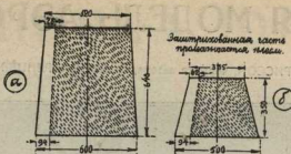
ТРУБЫ ФЮЗЕЛЯЖА В РАЗВЕРНУТОМ ВИДЕ (черт. 2). Они делаются из бумаги, вымоченной по форме трапеции: а — передняя часть, б — задняя часть. Защитные слои наклеиваются клеем.
