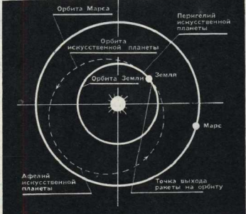
Расчетная орбита искусственной планеты относительно Солнца.
