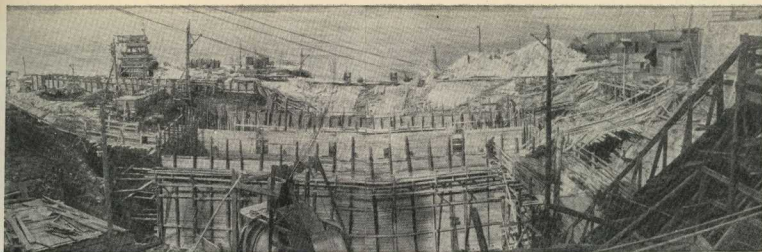
На строительстве ТЭЦ Куйбышевского гидроузла.
