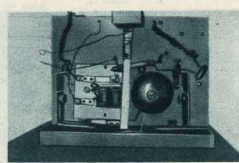
Грозозащитчик А. С. Попова (1895).
