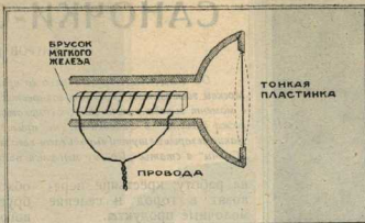
СХЕМА УСТРОЙСТВА ТЕЛЕФОННОГО АППАРАТА: от звуков слова тонкая пластина (мембрана) в трубке вибрирует и заставляет колебаться, вызывая в катушке электрические токи равной силы. Эти токи идут по проводам в аппарат слушающего и безаппарат магнитом находящийся там кусок железа, касаясь мембраны в точности как только колебания первой мембраны и, значит, воспроизводить слова, сказанные в первой аппарате
