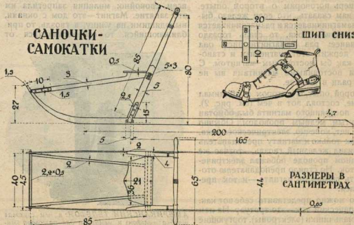
ЧЕРТЕЖИ САНОЧЕК-САМОКАТОК: вид сбоку, вид сверху и устройство шипа для ботинков.
