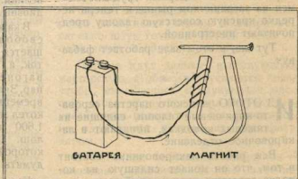
СПЛЕВА — Кусок мягкого железа становится магнитным и притягивает гвоздь, если по проводу будет идти электрический ток (рис. 1) СПРАВА — Если к постоянному магниту, обмотанному проводом, приблизить кусок железа, — в проводе возникнет электрический ток (рис. 2). В СЕРЕДИНЕ — РАЗРЕЗ ТЕЛЕФОННОЙ ТРУБКИ: S — магнитный стержень; C — железная пластинка (мембрана); D — проводочная обмотка; A и B — обжимной ободок трубки (рис. 3)
