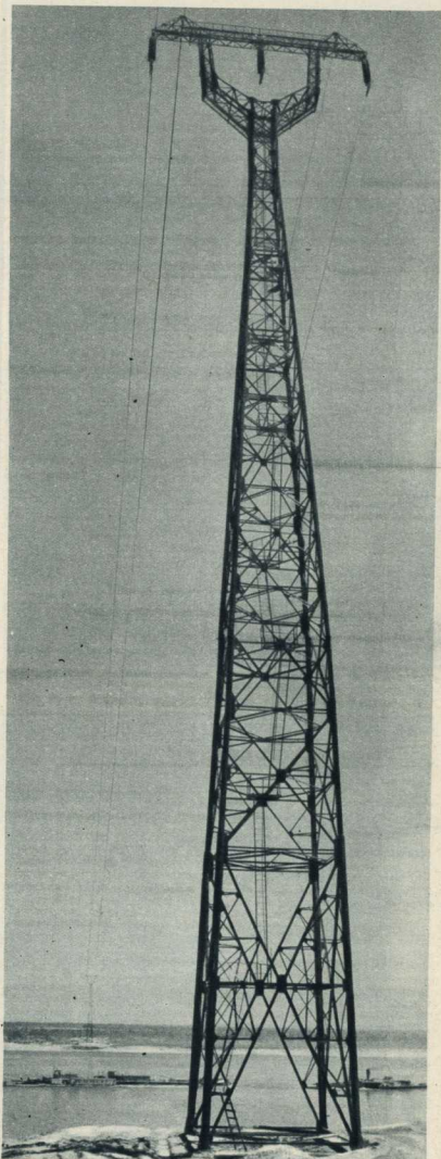
Сталинградгидрострой. 90-метровая переходная опора высоковольтной линии электропередачи через Волгу.
