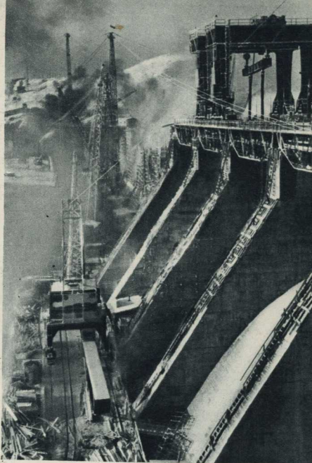
Водосливная плотина Усть-Каменогорской ГЭС.
