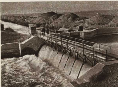
Гидротехнический узел в Вахшской долине.
