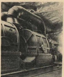
Паровая турбина высокого давления мощностью в 100 тысяч киловатт, изготовленная Ленинградским металлургическим заводом имени Сталина. Турбина предназначена для Сталинской ГРЭС, снабжающей электроэнергией Москву. Турбина сконструирована коллективом инженеров под руководством главного конструктора завода заслуженного Сталинской премии проф. М. И. Гринберга.
