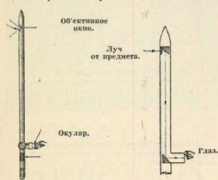
Рис. 1. Перископ типа «Разведчик».
