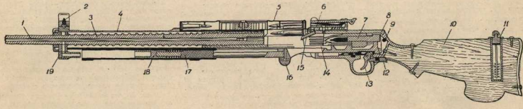
Вот как устроен ручной пулемет Дегтярева (разрез): 1) ствол, 2) мушка, 3) радиатор, 4) кожух, 5) магазин с патронами, 6) прицел, 7) ударник, 8) ствольная коробка, 9) замкатель, 10) приклад, 11) маеленка, 12) предохранитель, 13) спусковой крючок, 14) выбрасыватель стреляных гильз, 15) отражатель, 16) рукоятка рамы, 17) возвратная пружина, 18) поршень, 19) газовая камера.
