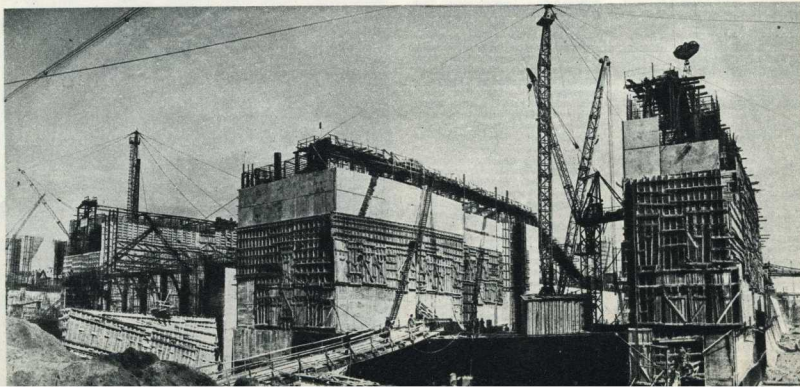
Бетонные работы на нижнем шлюзе — первом пусковом объекте Куйбышевгидростроя.
