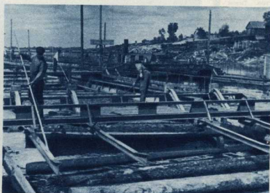
Весь добытый лес идёт к Волге, где мощные плотовальные машины собирают его в плоты. На снимке: момент сбора бревен плотовальной машиной.
