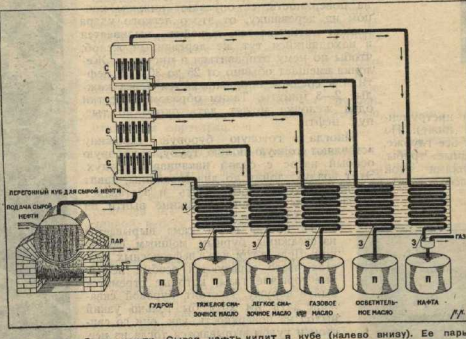
Схема переработки нефти. Сырая нефть кипит в кубе (наверху внизу). Ее пары, поднимаясь по трубе вверх, последовательно отходят по трубам направо и влево (3), помещенным в холодильниках (Х), чтобы затем унн в нижнем кубе снова кипела (4). Там получают тяжелые масла. Дальнейшая переработка состоит в том, что полученная в последнем кубе «мазута» поробным образом перегоняется в более легкие продукты, в том числе керосин и бензин
