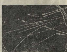
Фотография следа атомных частиц внутри «взрывной» камеры. Каждый след состоит из ивоннеств мелких водяных капелек (см. текст).
