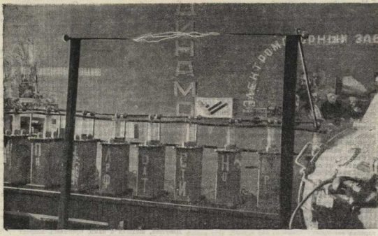
Украинский физико-технический институт работает сейчас над проблемой искусственного превращения элементов. Для этого превращения необходимо перестроить ядра атомов, что возможно только с помощью высоких электрических напряжений порядка сотен тысяч и миллионов вольт. Напряженье это может быть получено из первичного тока посредством его выпрявления через выпрявительную лампу (конкатер) и затем — многократным повышением напряжения в приборе, называемом генератором молний. Фото изображает установку генератора молний в Харькове. Между двумя проводниками проскакивает искра, представляющая собой искусственную молнию.
