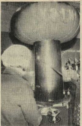
Высокие напряжения для превращения элементов можно также получать, накаливая большие электрические заряды на специальных проводниках (конденсаторах).
