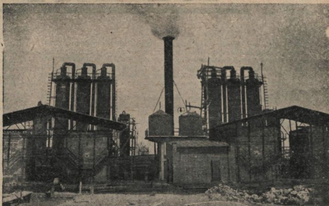
Советские трубчатые нефтеперерабатывающие заводы в Грозном.
