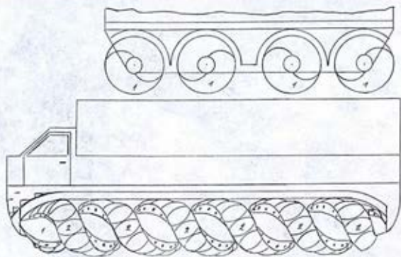
Роликовый шнекоход.
