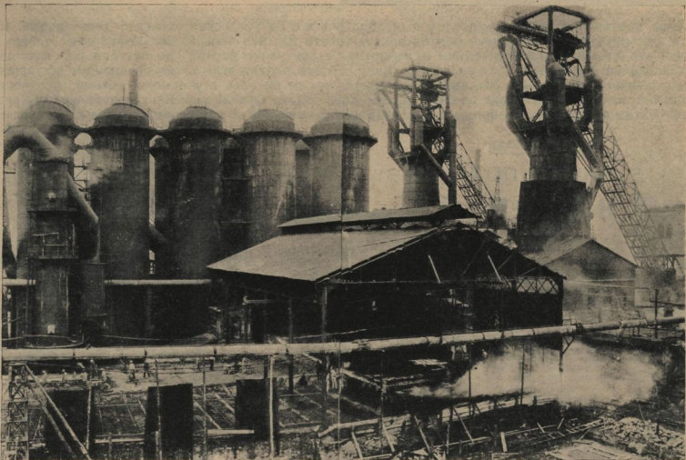
Керченский чугунолитейный завод. Общий вид.
