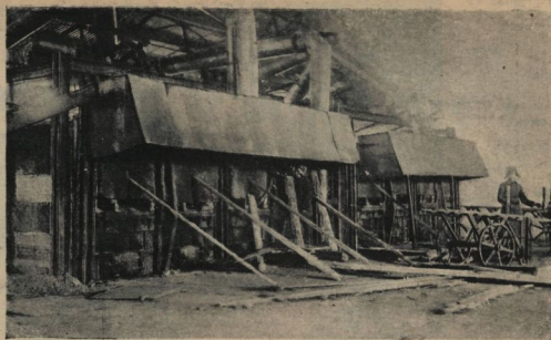
ТАГИЛ. Оборудование печей в новом листообойном цехе.
