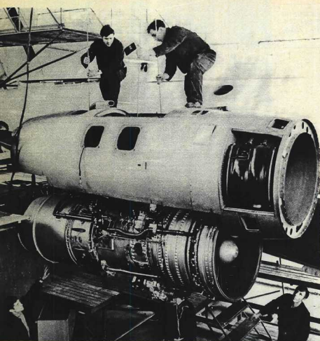
ИДЕТ МОНТАЖ ДВИГАТЕЛЕЙ.
