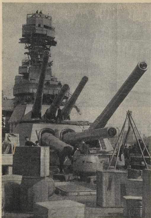
Боевая мощь и ее башни с 16-ми дюймовыми орудиями. Стреляет на 40 километров, снаряд в 60 пудов.
