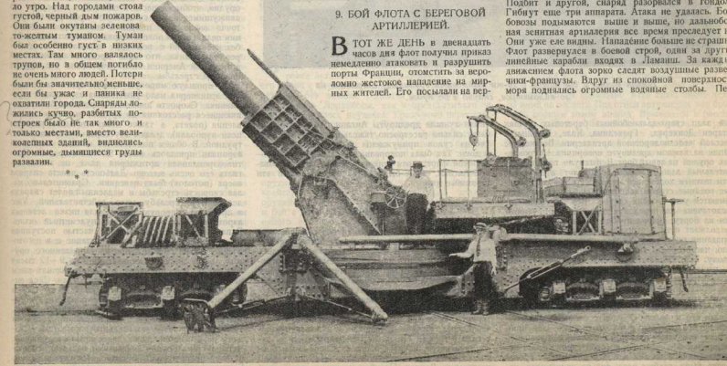
Здесь изображена 16" глубина, стреляющая на 22 километра — снарядом в 60 фундов. Война создала новый род тяжелой артиллерии, установленной на железнодорожных платформах.
