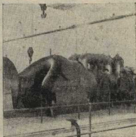
РОТОР ГЕНЕРАТОРА 4-х ТУРБИНЫ ДНЕПРОПЕТРОВСКОЙ ЭЛЕКТРОСТАНЦИИ В СБОРКЕ.
