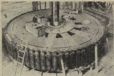
РОТОР ГЕНЕРАТОРА 4-х ТУРБИНЫ ДНЕПРОПЕТРОВСКОЙ ЭЛЕКТРОСТАНЦИИ В СБОРКЕ.
