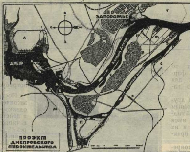
ДНЕПРОСТРОЙ: а) плотина, б) станция, в) разгрузочный канал, г) нефтяная канализация, д) шлюзы, е) заросшая плотина, ж) затопляемая плотина, з) устьевая плотина, и) судостроительный завод, к) маяк и размытый базис, л) аэропортный завод, м) нефтезавод, н) верхний взлет, о) нижний взлет, п) коллельная канализация, р) турбина, с) водозабор Юзовских, т) фабрично-заводской район.
